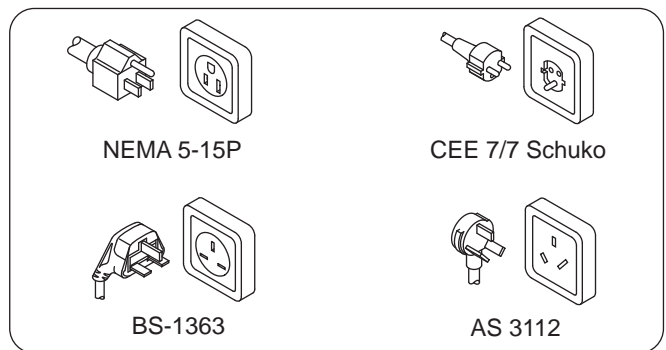
Steckerkonfigurationen
